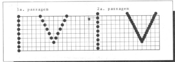
Figura 4 — Formação de caráter em matriz de ponto de 18 x 40.
